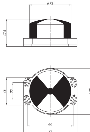
Индикатор-семафор
