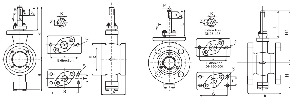
Размеры, мм Межфланцевое соединение
