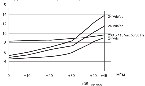
с крутящий момент/время поворота на 90°
