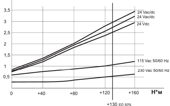
А крутящий момент/потребление
