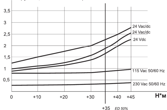
А крутящий момент/потребление
