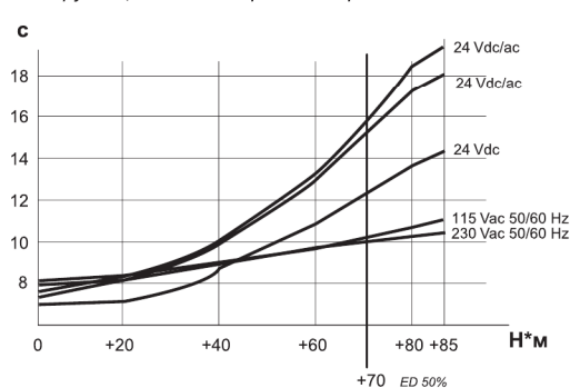
с крутящий момент/время поворота на 90°
