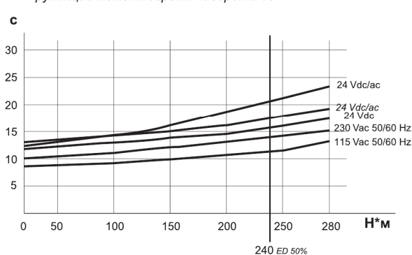
Б крутящий момент /время поворота 90°
